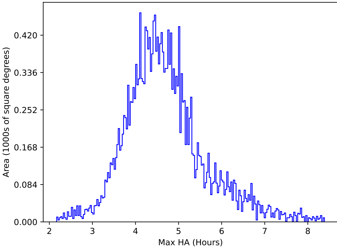
too_ignore_10_4v3.4_10yrs All sky y band: Max HA
