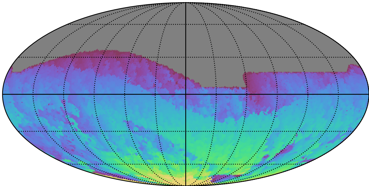
too_ignore_10_4v3.4_10yrs All sky i band: Max HA
