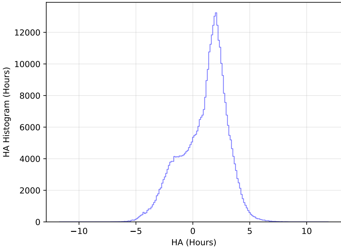
too_ignore_10_4v3.4_10yrs All sky y band: HA Histogram
