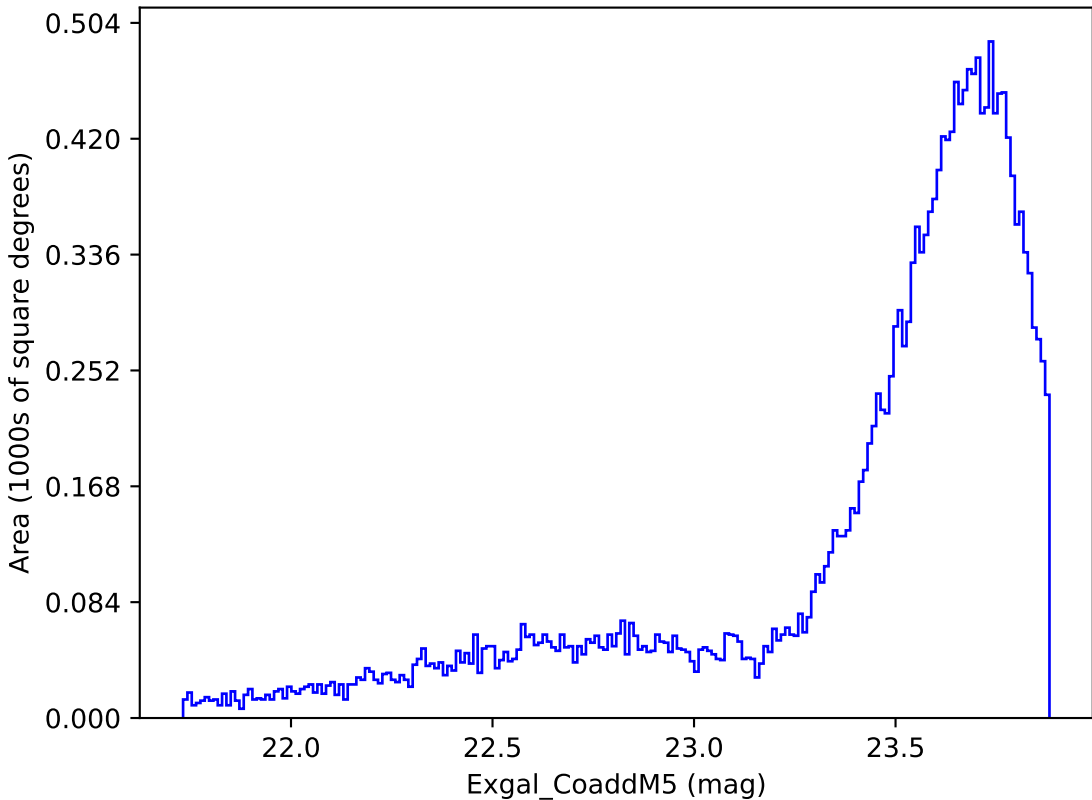
too_ignore_10_4v3.4_10yrs Yr 1 y band: Exgal_CoaddM5
