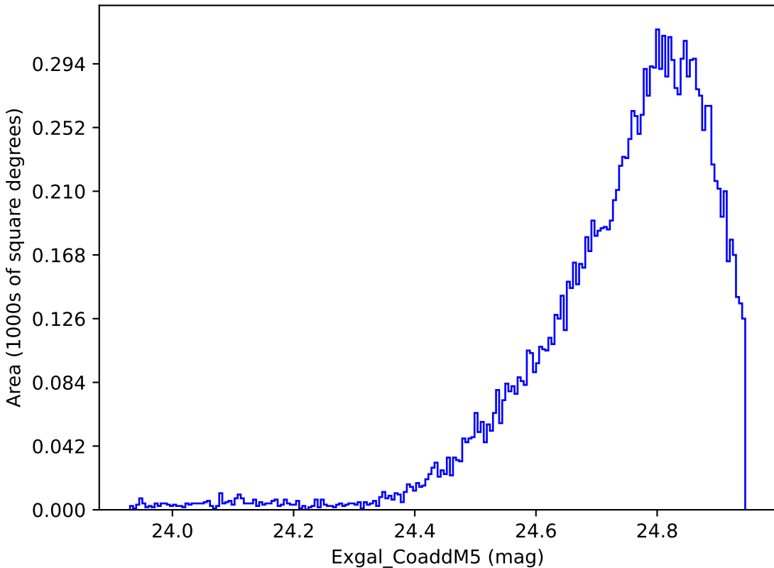
too_ignore_10_4v3.4_10yrs WFD y band: Exgal_CoaddM5
