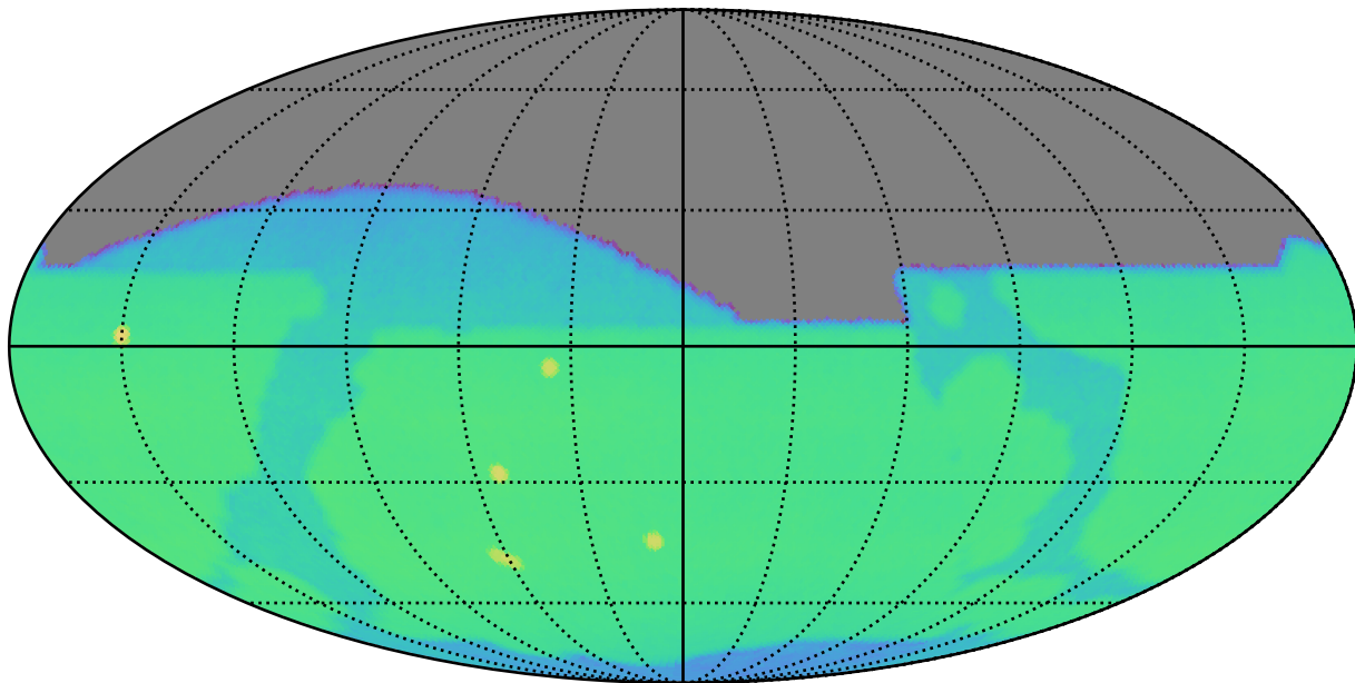
too_ignore_10_4v3.4_10yrs i: CoaddM5
