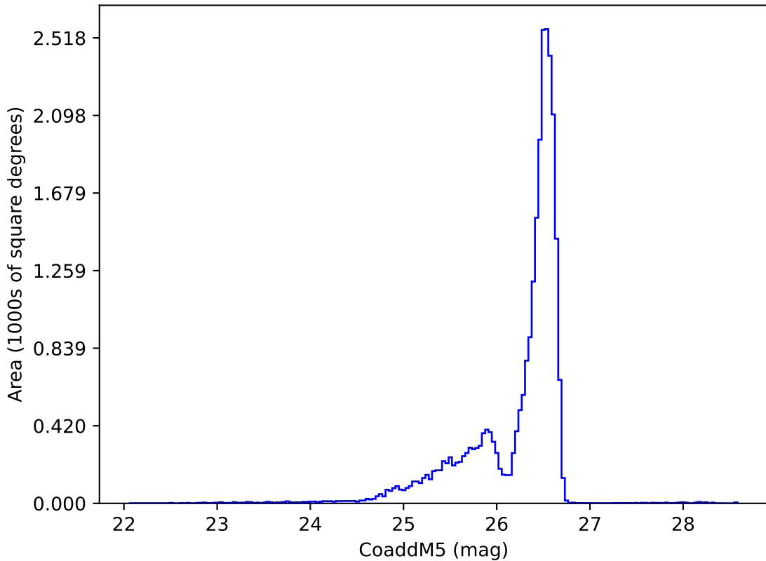
too_ignore_10_4v3.4_10yrs i: CoaddM5
