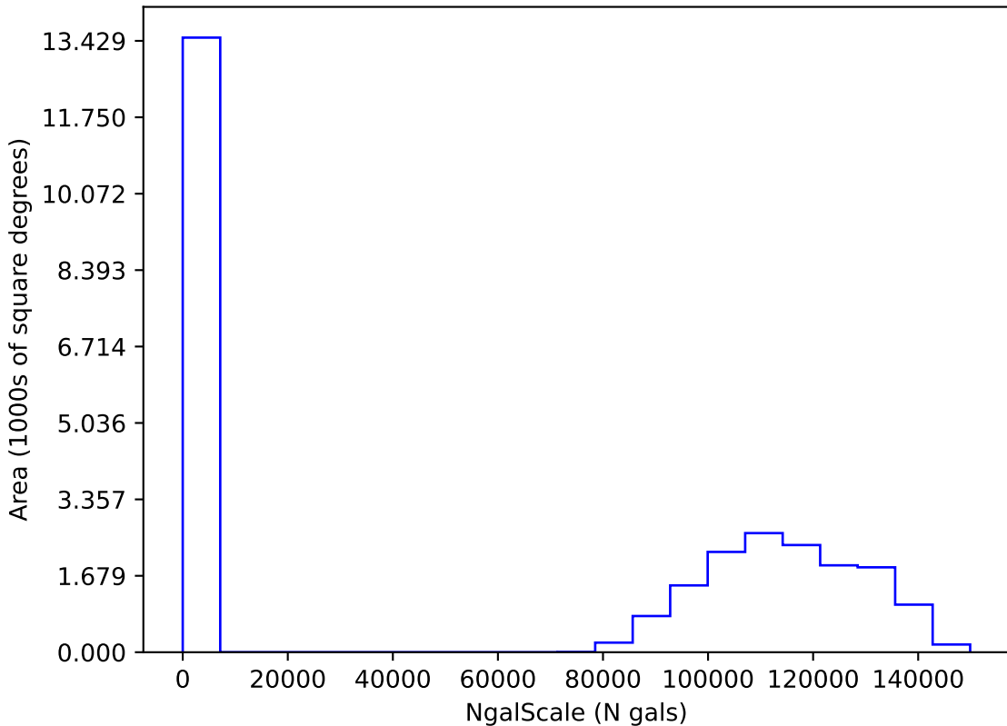
too_ignore_10_1v3.4_10yrs i: NgalScale
