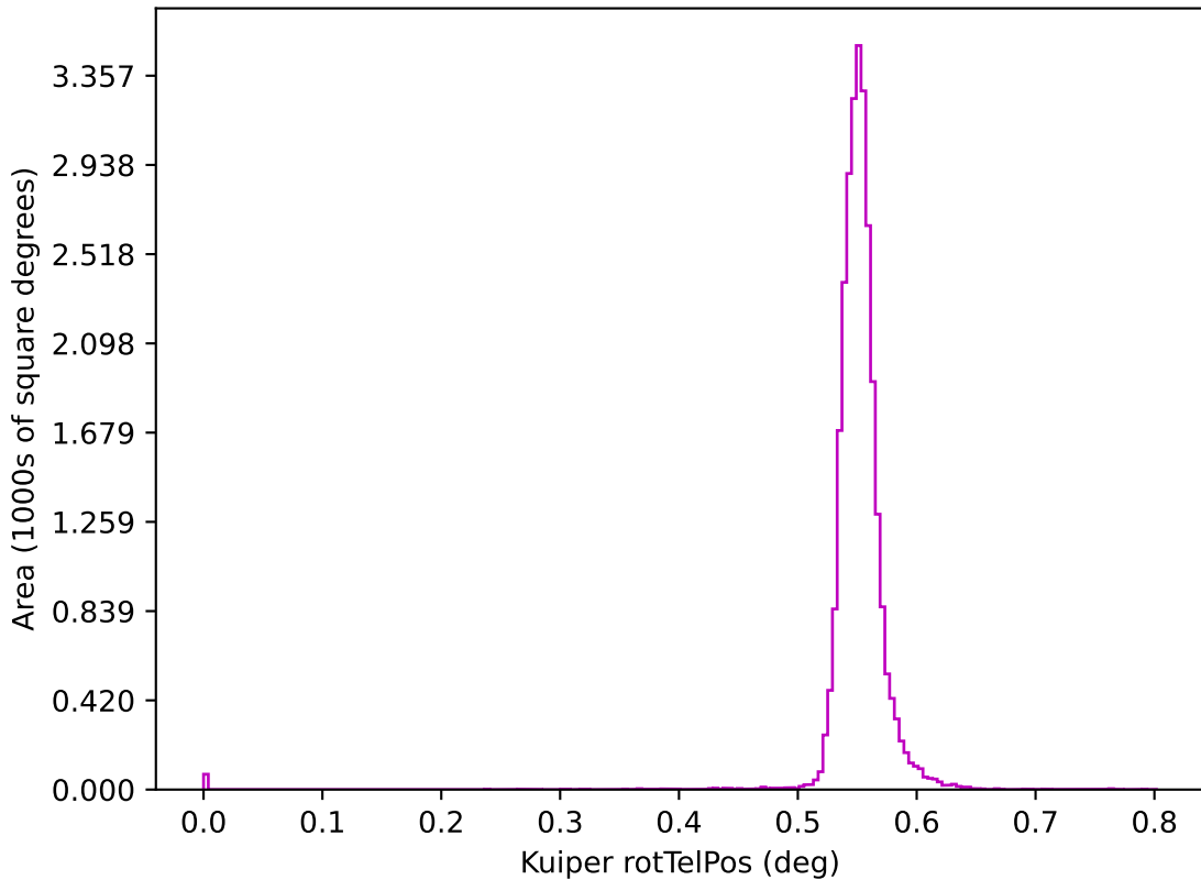
too_ignore_10_1v3.4_10yrs z: Kuiper rotTelPos
