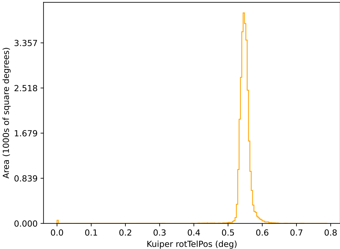
too_ignore_10_1v3.4_10yrs r: Kuiper rotTelPos
