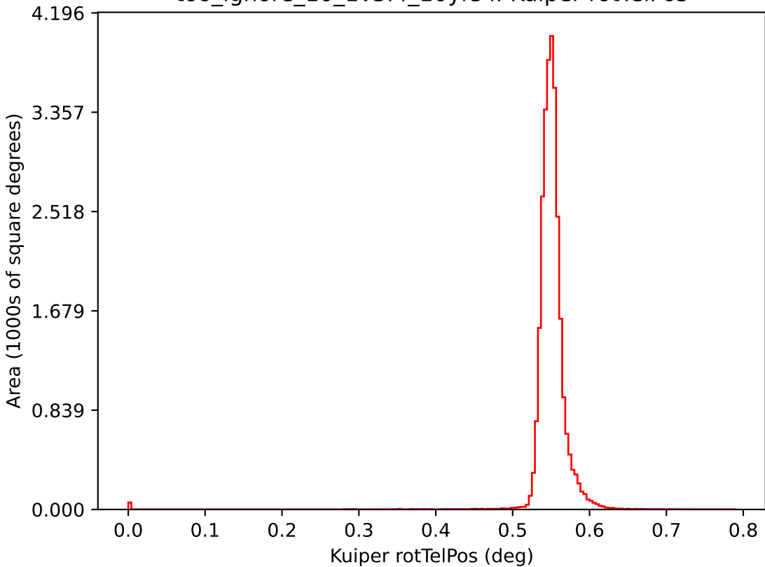
too_ignore_10_1v3.4_10yrs i: Kuiper rotTelPos
