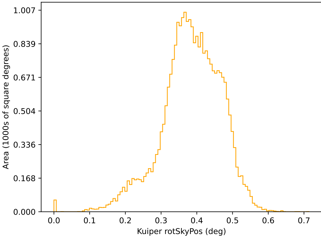
too_ignore_10_1v3.4_10yrs r: Kuiper rotSkyPos
