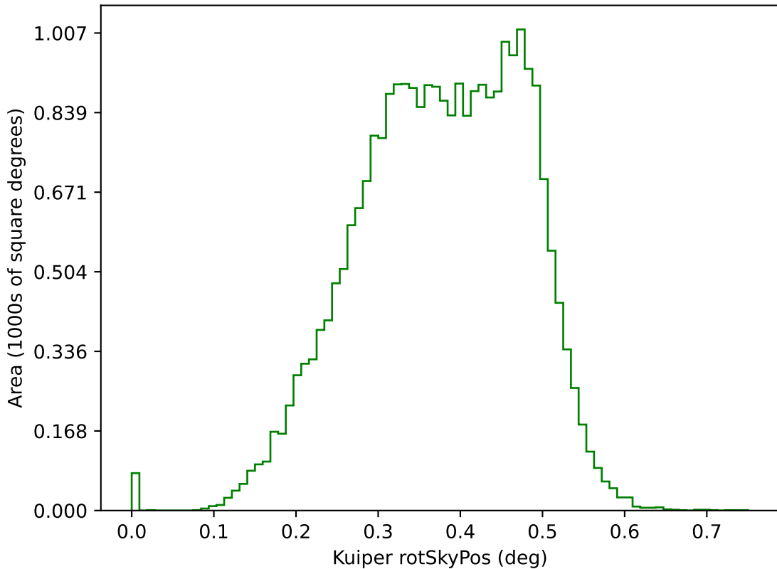
too_ignore_10_1v3.4_10yrs g: Kuiper rotSkyPos
