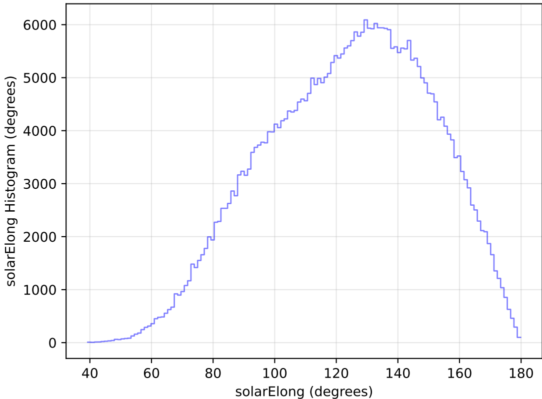
too_ignore_10_1v3.4_10yrs All sky y band: solarElong Histogram
