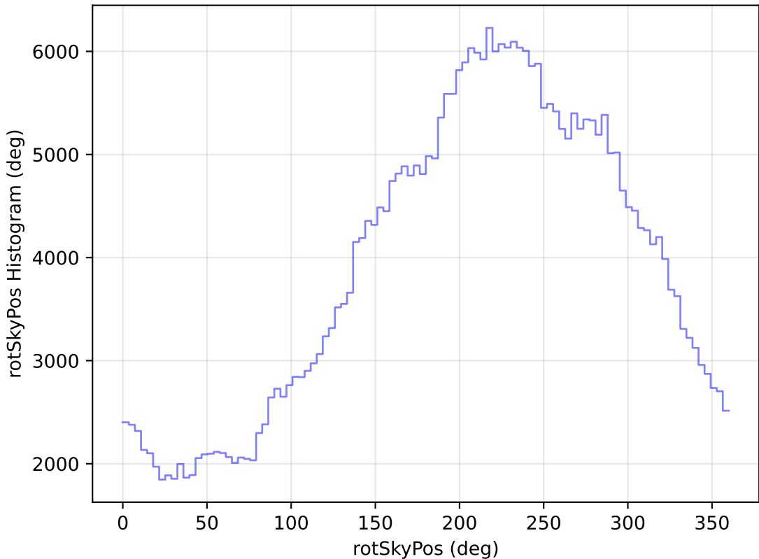
too_ignore_10_1v3.4_10yrs WFD y band: rotSkyPos Histogram
