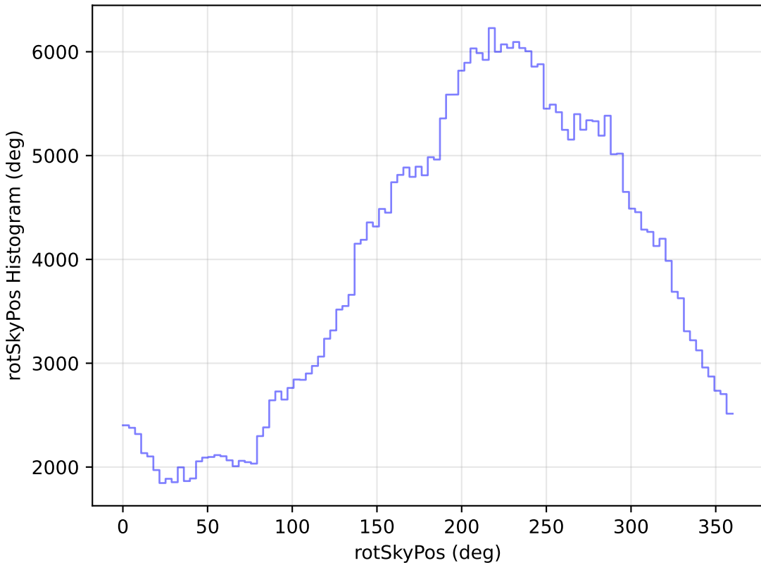
too_ignore_10_1v3.4_10yrs All sky y band: rotSkyPos Histogram
