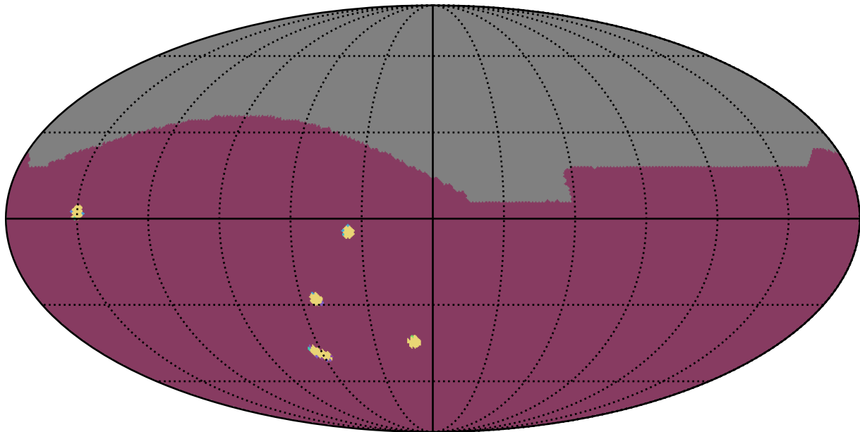
too_ignore_10_1v3.4_10yrs All sky: NumberOfQuickRevisits
