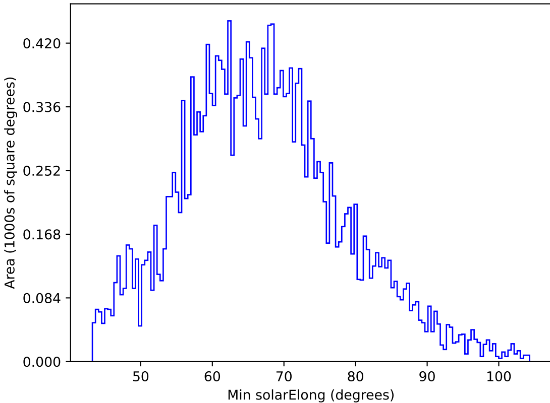
too_ignore_10_1v3.4_10yrs All sky y band: Min solarElong
