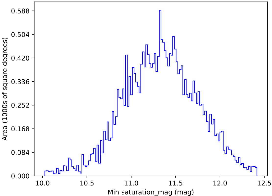
too_ignore_10_1v3.4_10yrs All sky y band: Min saturation_mag
