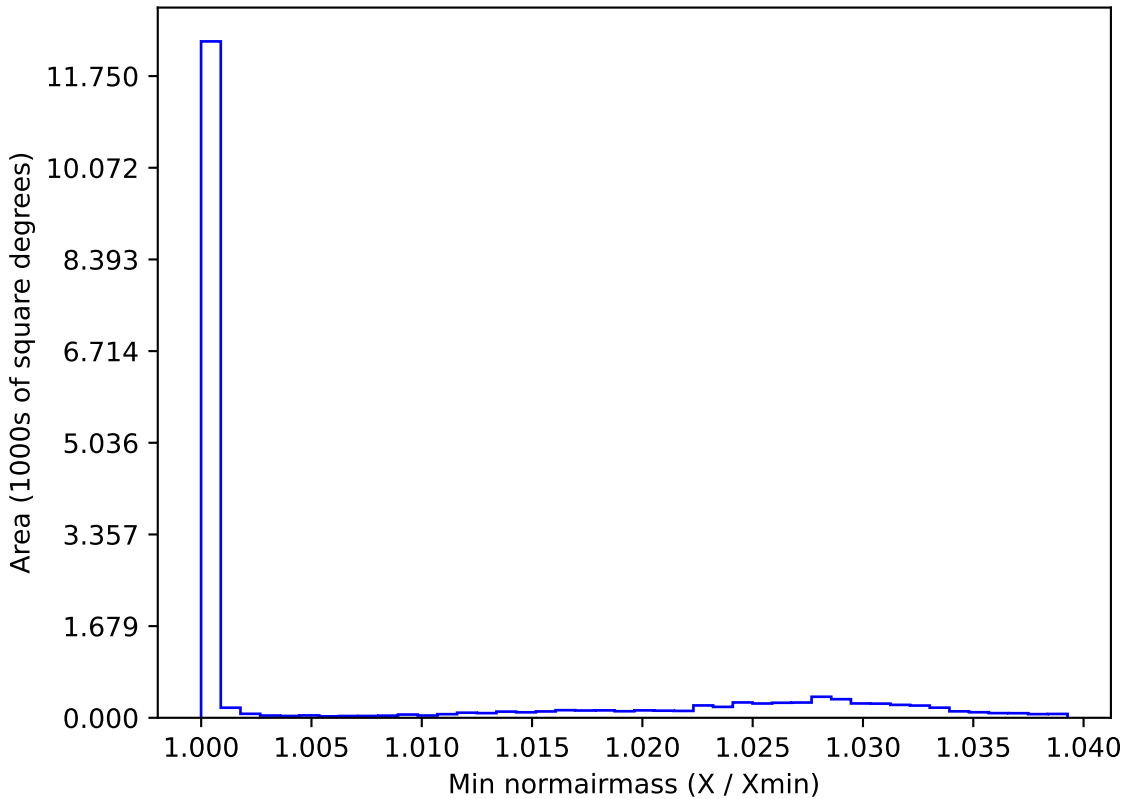
too_ignore_10_1v3.4_10yrs WFD y band: Min normairmass
