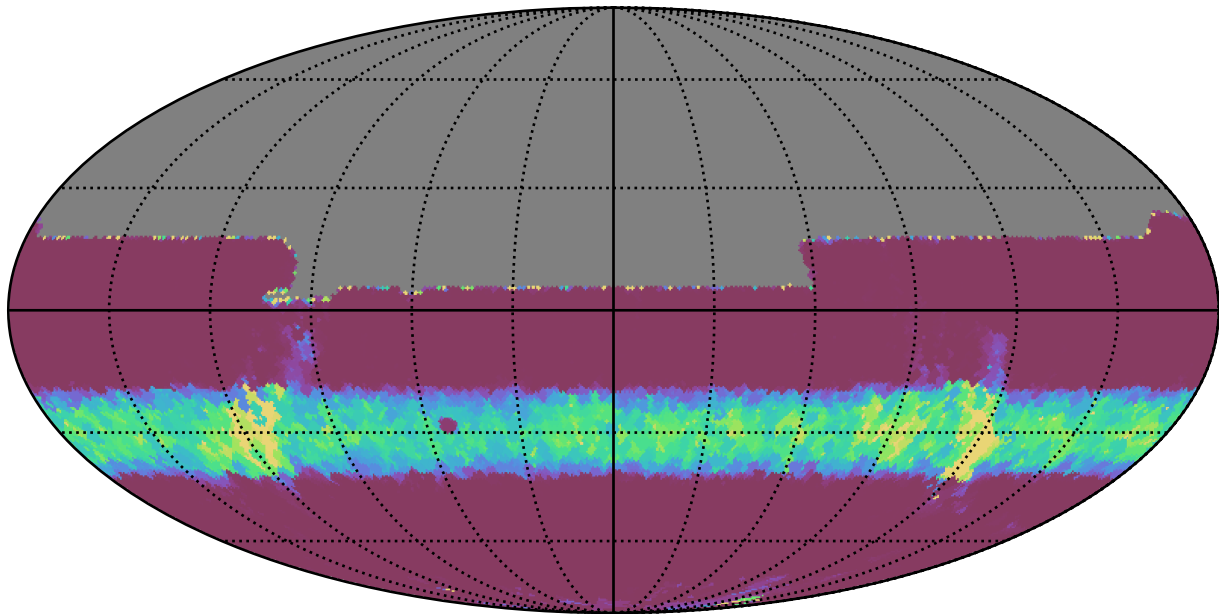
too_ignore_10_1v3.4_10yrs All sky y band: Min normairmass
