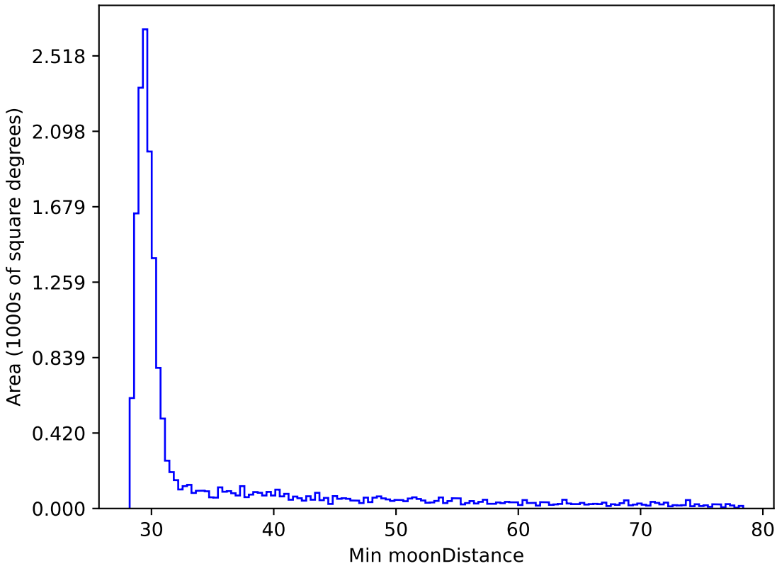
too_ignore_10_1v3.4_10yrs WFD y band: Min moonDistance
