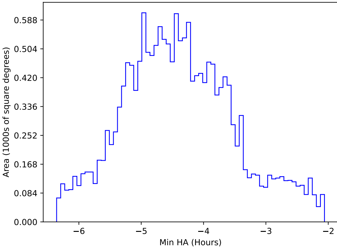
too_ignore_10_1v3.4_10yrs WFD z band: Min HA
