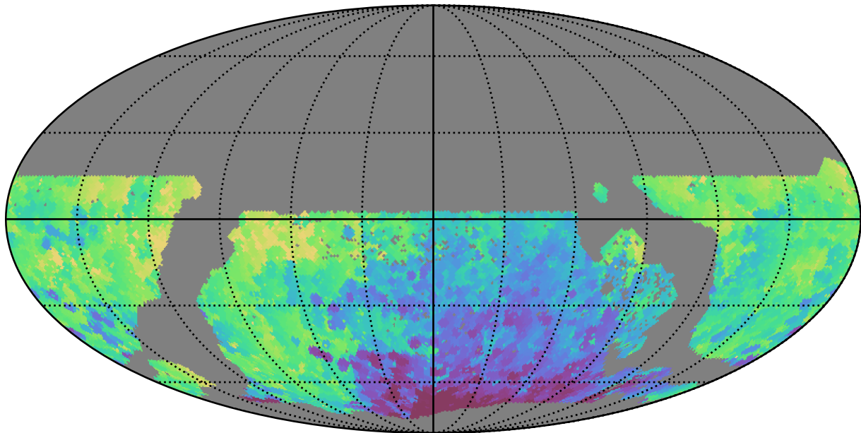
too_ignore_10_1v3.4_10yrs WFD y band: Min HA
