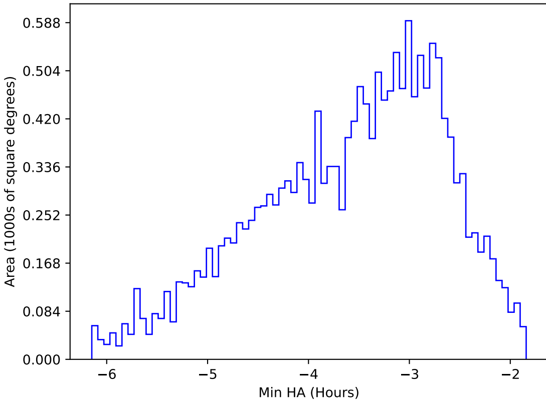
too_ignore_10_1v3.4_10yrs WFD y band: Min HA
