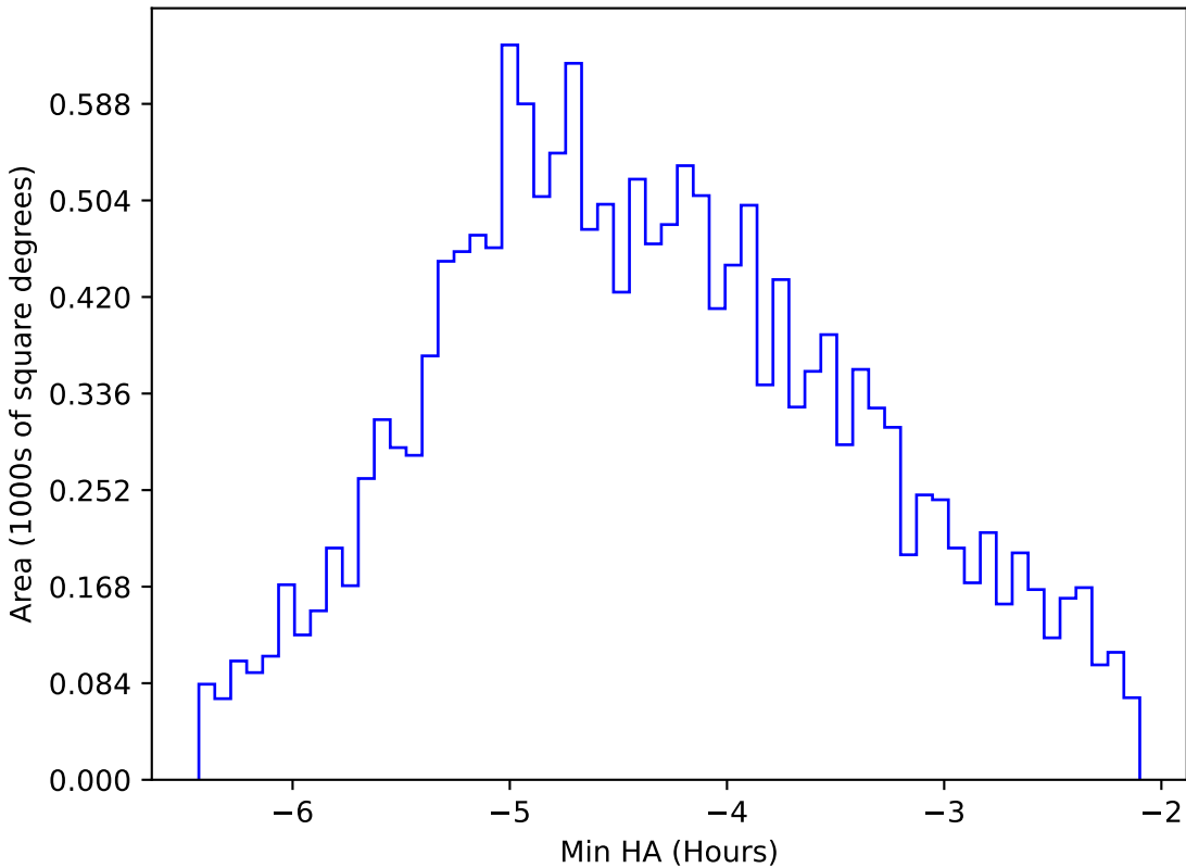
too_ignore_10_1v3.4_10yrs WFD i band: Min HA
