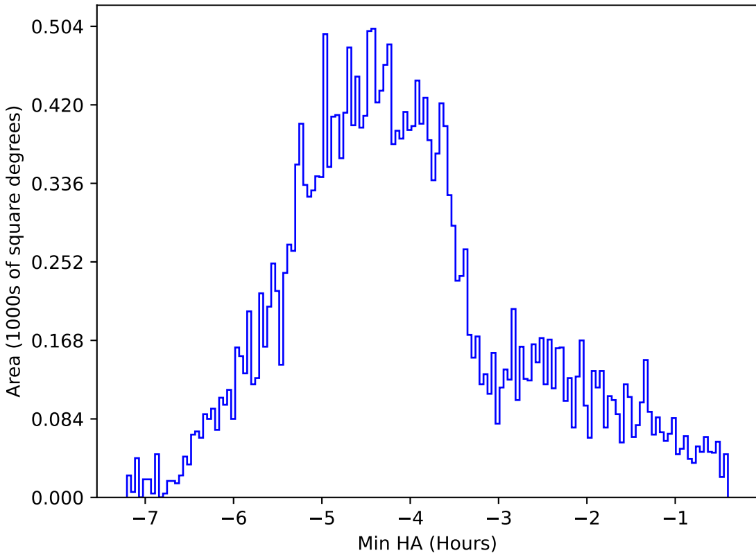
too_ignore_10_1v3.4_10yrs All sky z band: Min HA
