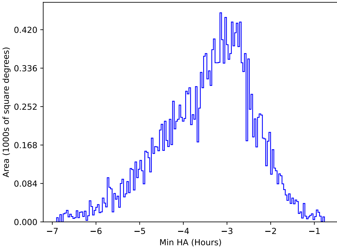
too_ignore_10_1v3.4_10yrs All sky y band: Min HA
