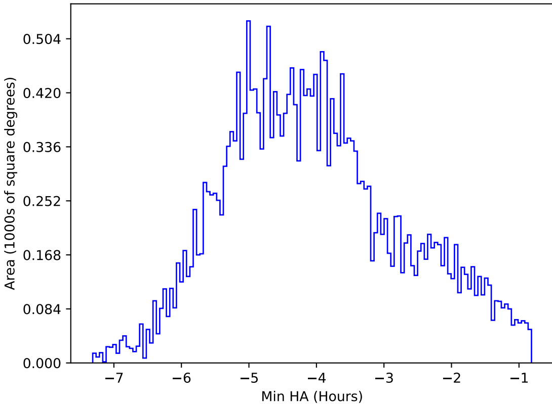
too_ignore_10_1v3.4_10yrs All sky i band: Min HA
