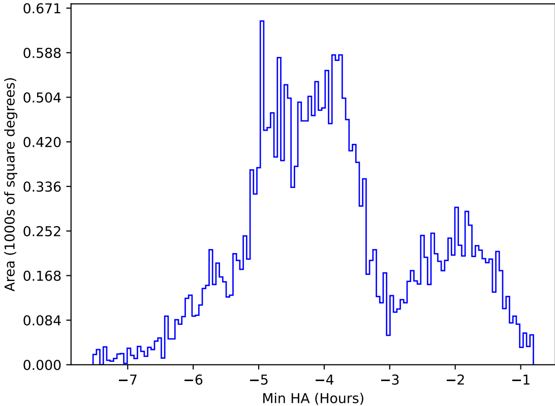
too_ignore_10_1v3.4_10yrs All sky g band: Min HA
