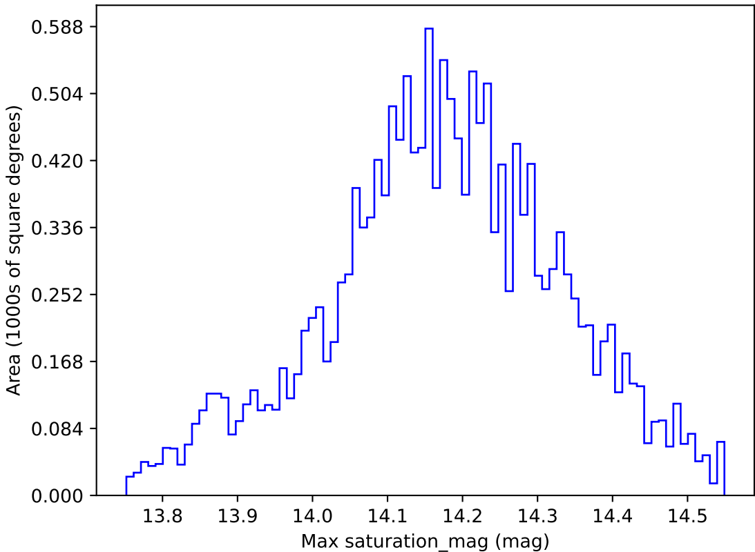
too_ignore_10_1v3.4_10yrs WFD y band: Max saturation_mag
