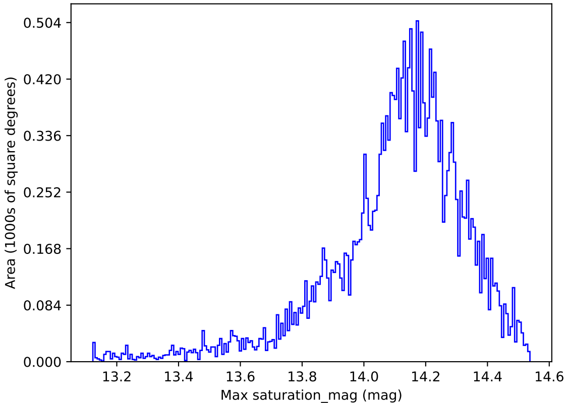
too_ignore_10_1v3.4_10yrs All sky y band: Max saturation_mag
