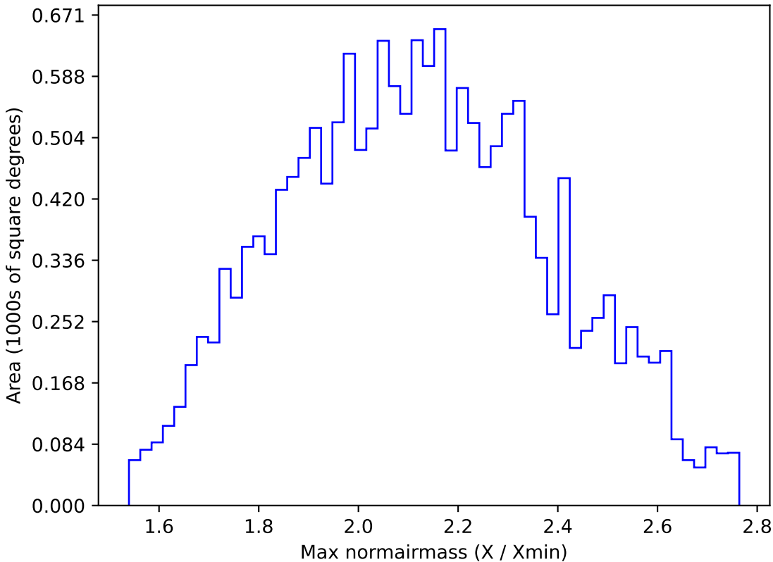
too_ignore_10_1v3.4_10yrs WFD y band: Max normairmass
