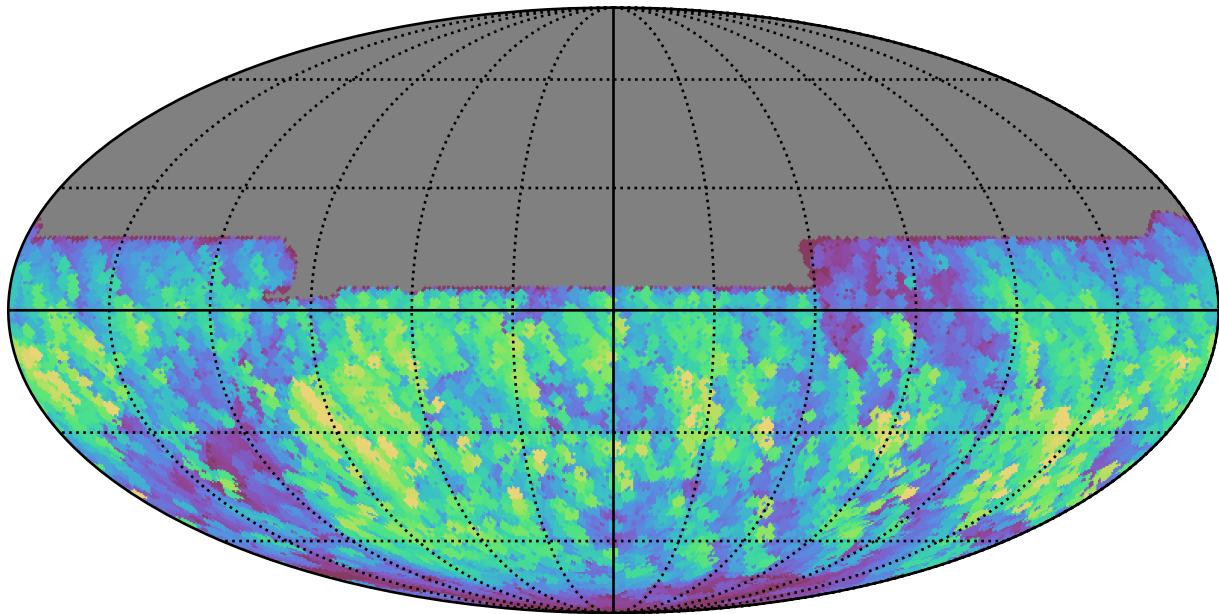
too_ignore_10_1v3.4_10yrs All sky y band: Max normairmass
