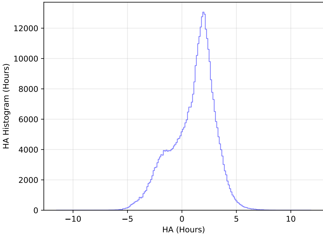
too_ignore_10_1v3.4_10yrs All sky y band: HA Histogram
