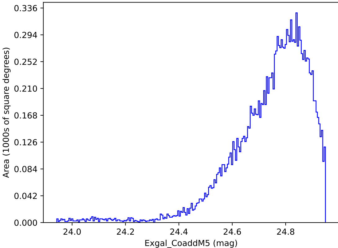
too_ignore_10_1v3.4_10yrs WFD y band: Exgal_CoaddM5
