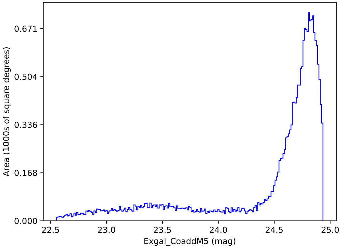
too_ignore_10_1v3.4_10yrs All sky y band: Exgal_CoaddM5
