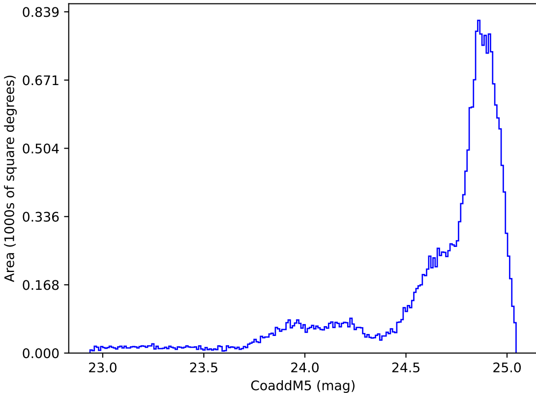
too_ignore_10_1v3.4_10yrs All sky y band: CoaddM5
