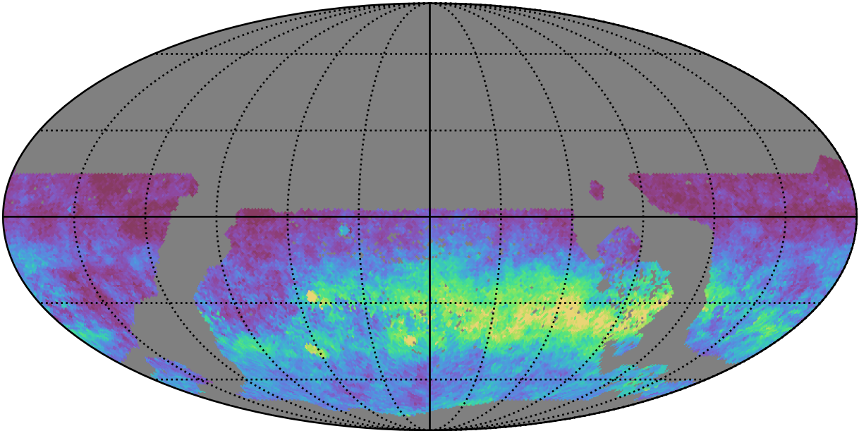
too_ignore_10_1v3.4_10yrs WFD y band: AngleRms rotSkyPos
