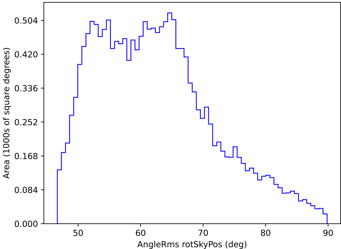
too_ignore_10_1v3.4_10yrs WFD y band: AngleRms rotSkyPos
