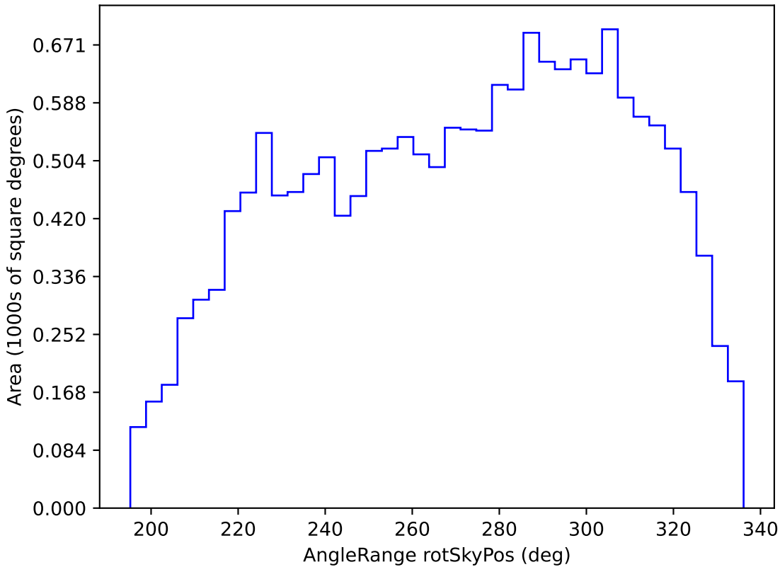
too_ignore_10_1v3.4_10yrs WFD y band: AngleRange rotSkyPos
