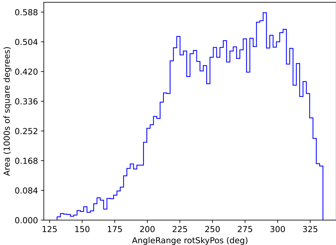
too_ignore_10_1v3.4_10yrs All sky y band: AngleRange rotSkyPos
