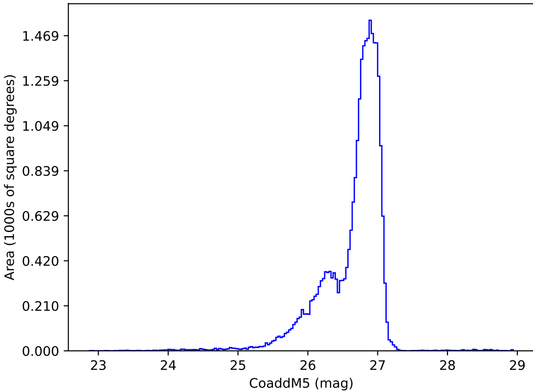
too_ignore_10_1v3.4_10yrs g: CoaddM5
