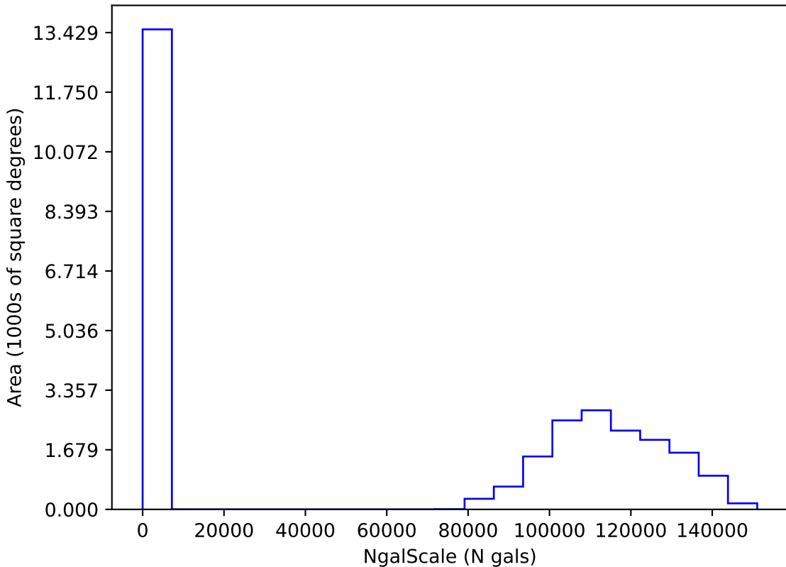
too_ignore_100_4v3.4_10yrs i: NgalScale
