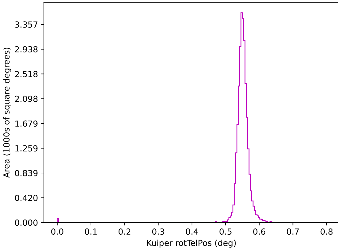
too_ignore_100_4v3.4_10yrs z: Kuiper rotTelPos
