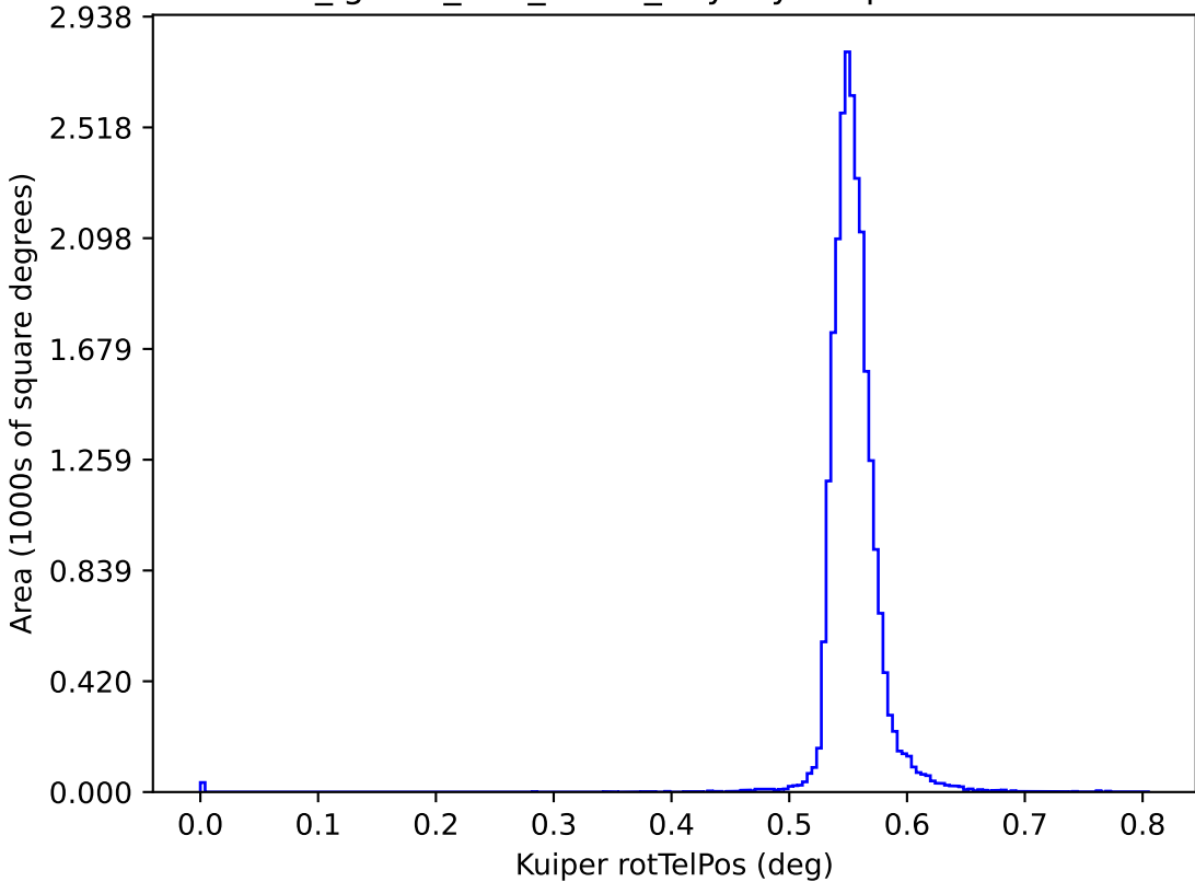
too_ignore_100_4v3.4_10yrs y: Kuiper rotTelPos
