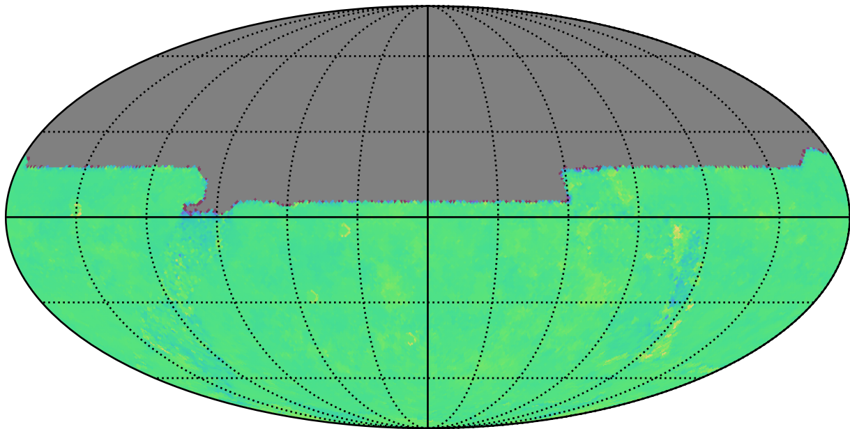
too_ignore_100_4v3.4_10yrs u: Kuiper rotTelPos
