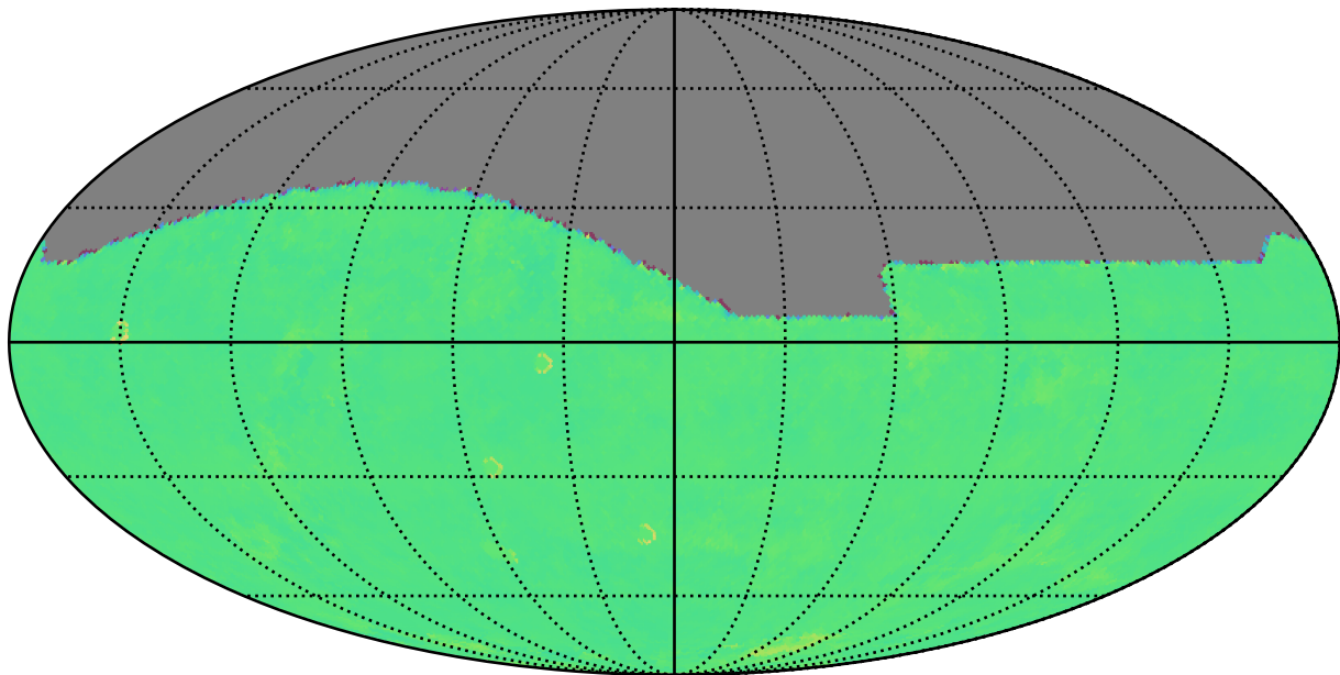
too_ignore_100_4v3.4_10yrs r: Kuiper rotTelPos
