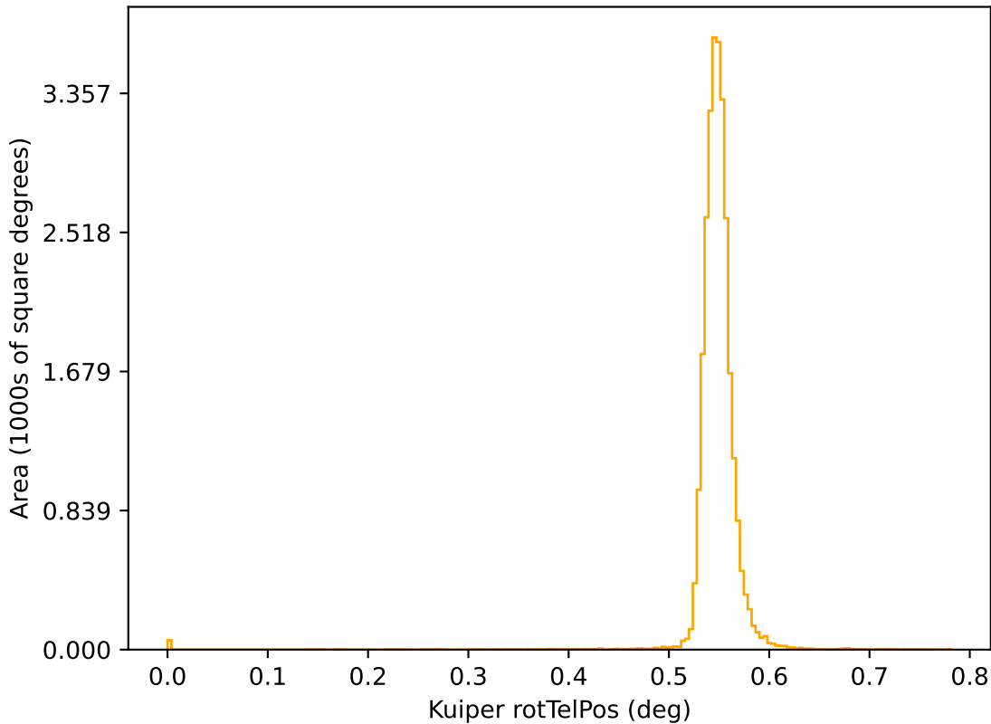
too_ignore_100_4v3.4_10yrs r: Kuiper rotTelPos
