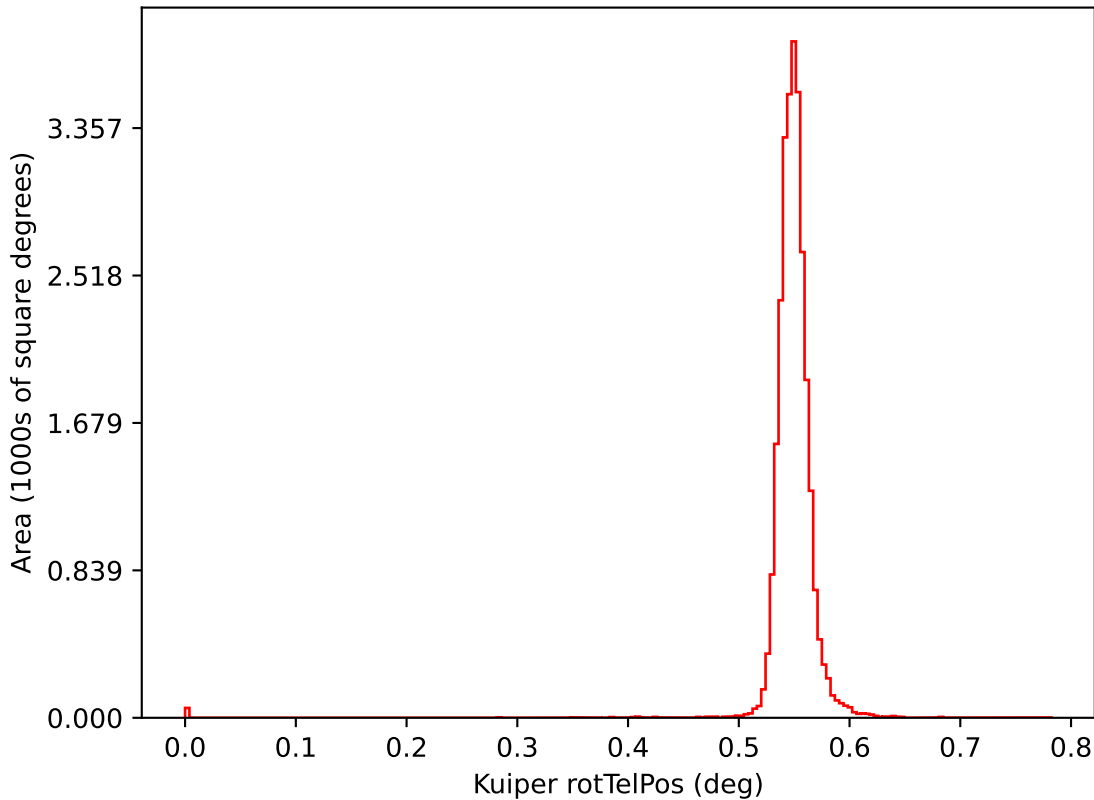
too_ignore_100_4v3.4_10yrs i: Kuiper rotTelPos
